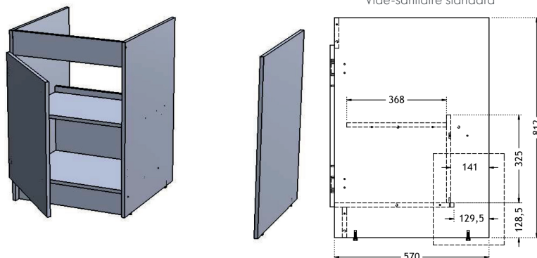
VUE DE DROITE Vide-sanitaire standard
